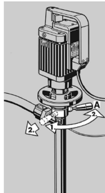
obr. 6 Rura pompy RE SS /
