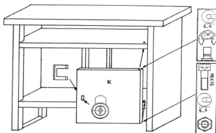
Montaż szuflady
